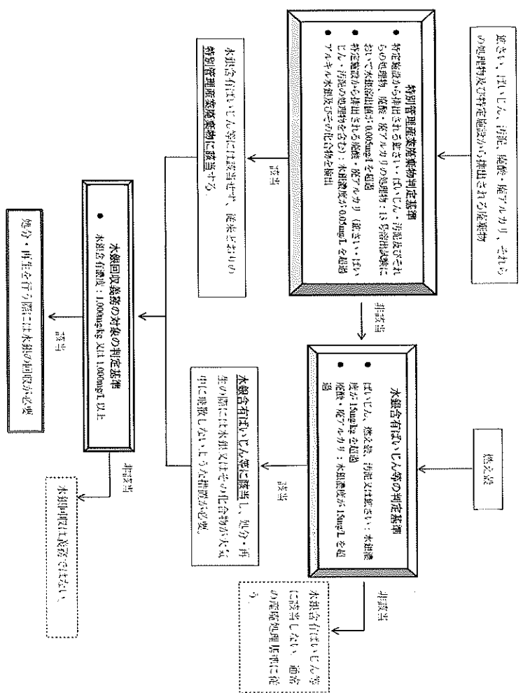
図 4.1.1 水銀汚染物の分類及び必要な措置
