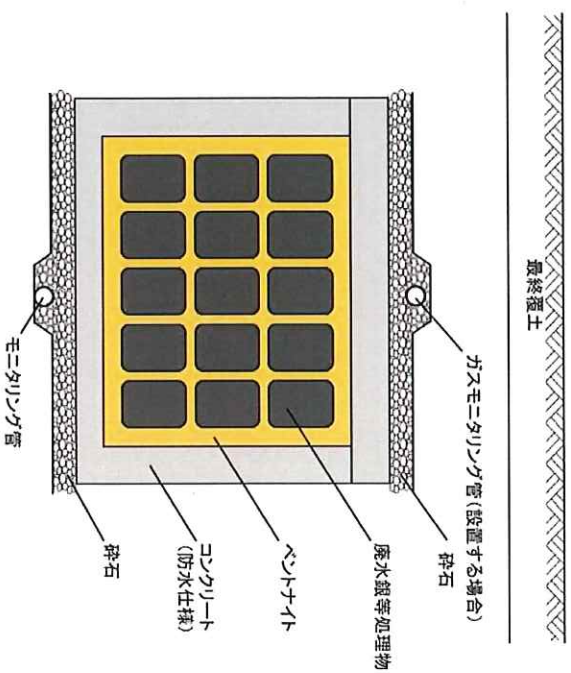
図 3.7.4 廃水銀等処理物の雨水浸入防止措置の例
