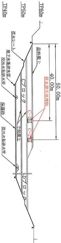
図 3.7.9 埋め立てた廃水銀等処理物の埋立位置の記録例 (a-a 断面図)
